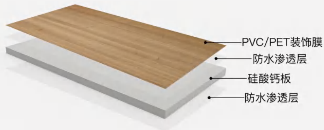
- PVC/PET平贴板 -
