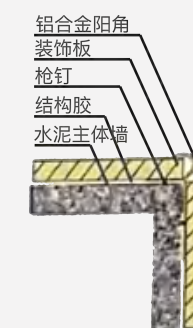
阳角工艺
