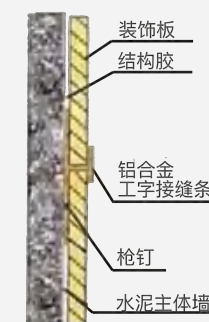
工字接缝条
