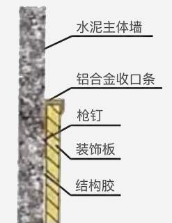
侧边收口
