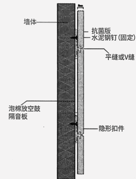
干挂式安装示意图
