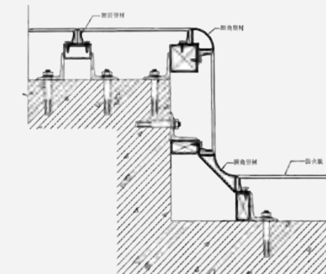
安装示意图
